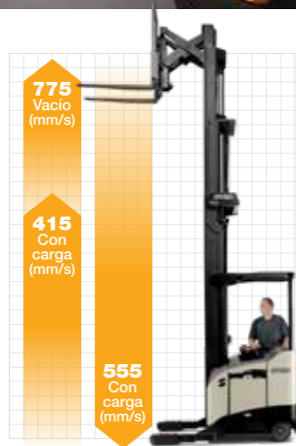
Levante Descenso (Sistema hidráulico AC)
